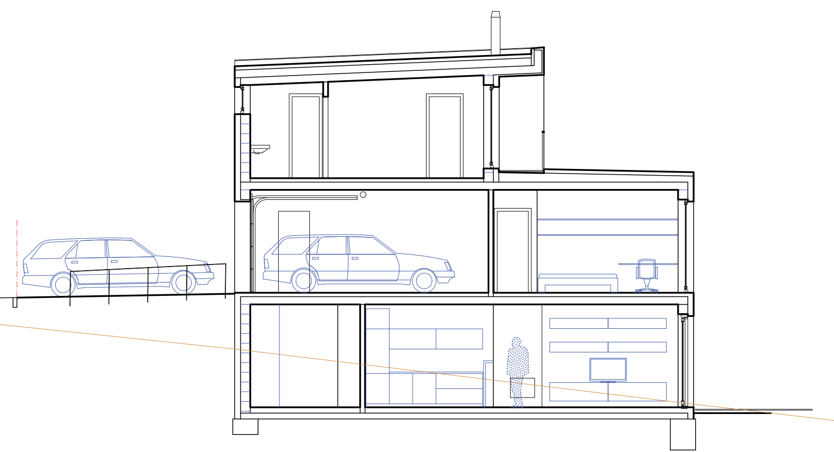
řez příčný
